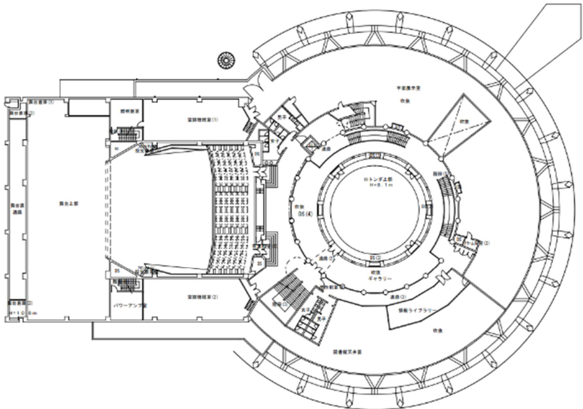
2 階平面図
