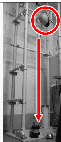
衝撃吸収性試験の様子
